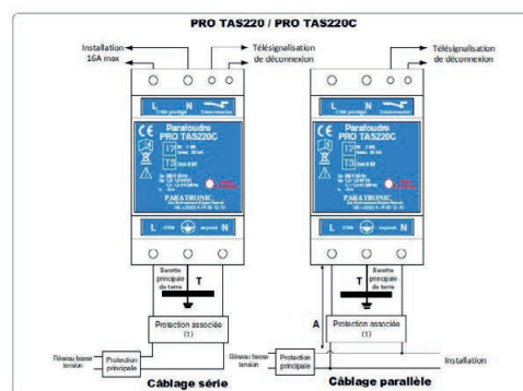
Schéma de raccordement du PRO TAS220C
