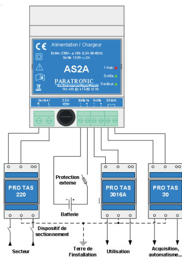
Schéma de raccordement AS2A
